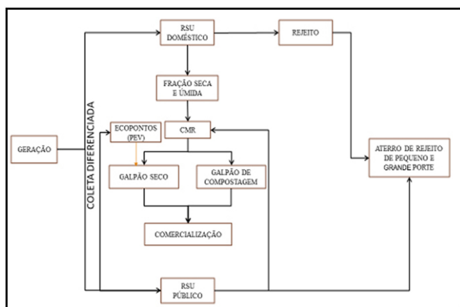
Figura 18 – Rota tecnológica dos Resíduos Sólidos Urbanos da Região do Sertão Central
